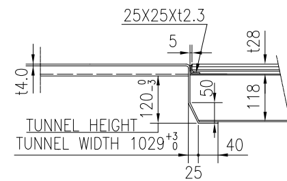
SECTION D-D 1:5
